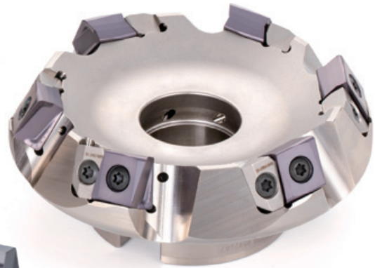
TGM16**SA APMX 12.4 mm 60° Fräser
