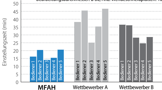
Der MFAH kann die Rüstzeiten deutlich verkürzen
