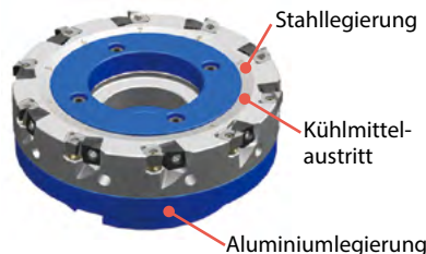
Leichter Hybridkörper ø 80 mm – ø 315 mm
