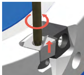
Einzigartige Konstruktion zur problemlosen Einstellung an der Stirnseite
